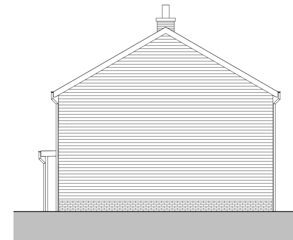
Right Elevation 1 : 100
