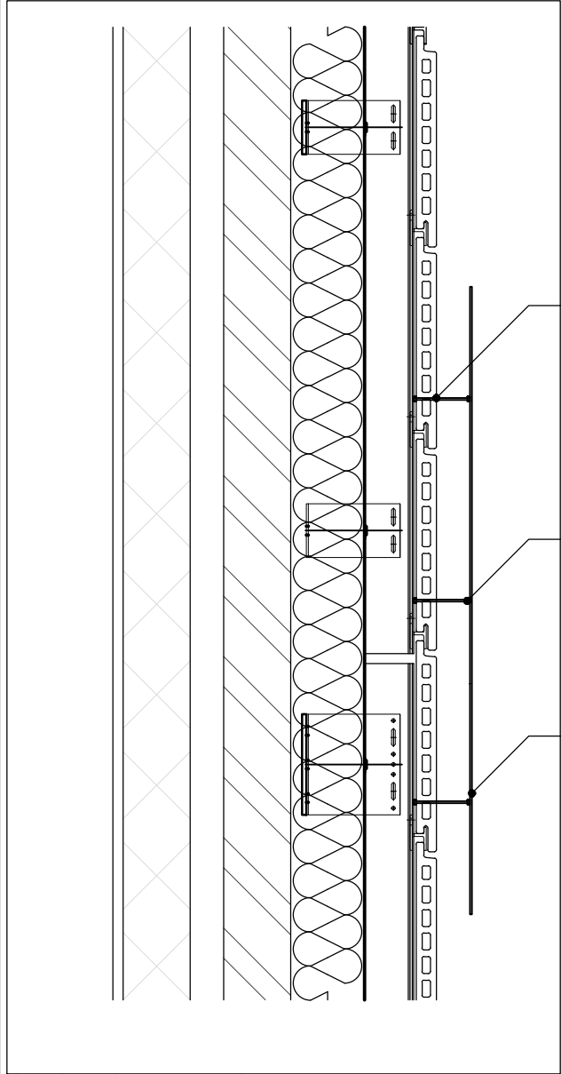
SECTION A-A @1:10
