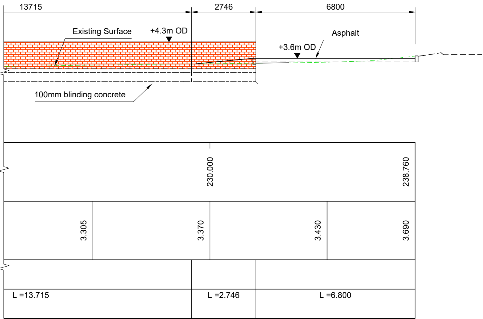
Elevation 1:100
